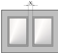
Dubbelmontage x=100mm
